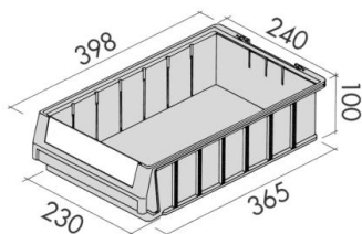
Kuweta magazynowa 400 x 240 x 100mm
