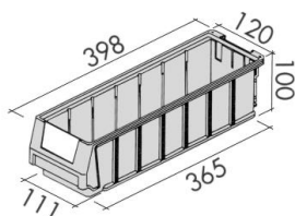
Kuweta magazynowa 400 x 120 x 100mm
