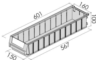
Kuweta magazynowa 600 x 160 x 100mm
