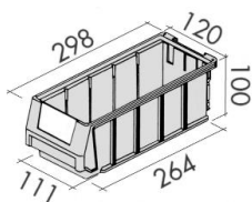
Kuweta magazynowa 300 x 120 x 100mm
