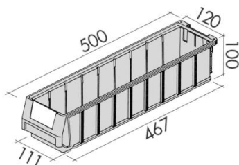
Kuweta magazynowa 500 x 120 x 100mm
