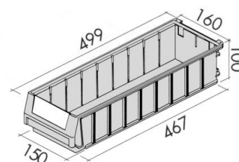
Kuweta magazynowa 500 x 160 x 100mm
