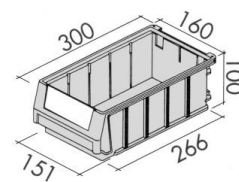
Kuweta magazynowa 300 x 160 x 100mm
