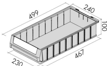
Kuweta magazynowa 500 x 240 x 100mm
