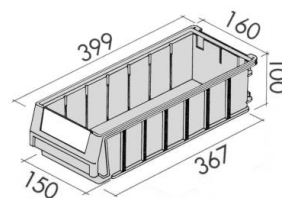
Kuweta magazynowa 400 x 160 x 100mm
